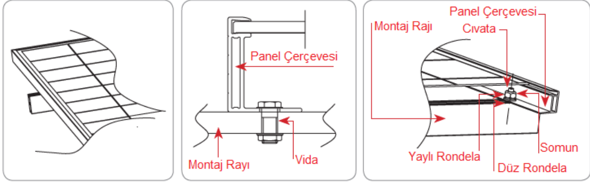
Şekil 2: Montaj deliklerine göre kurulum
