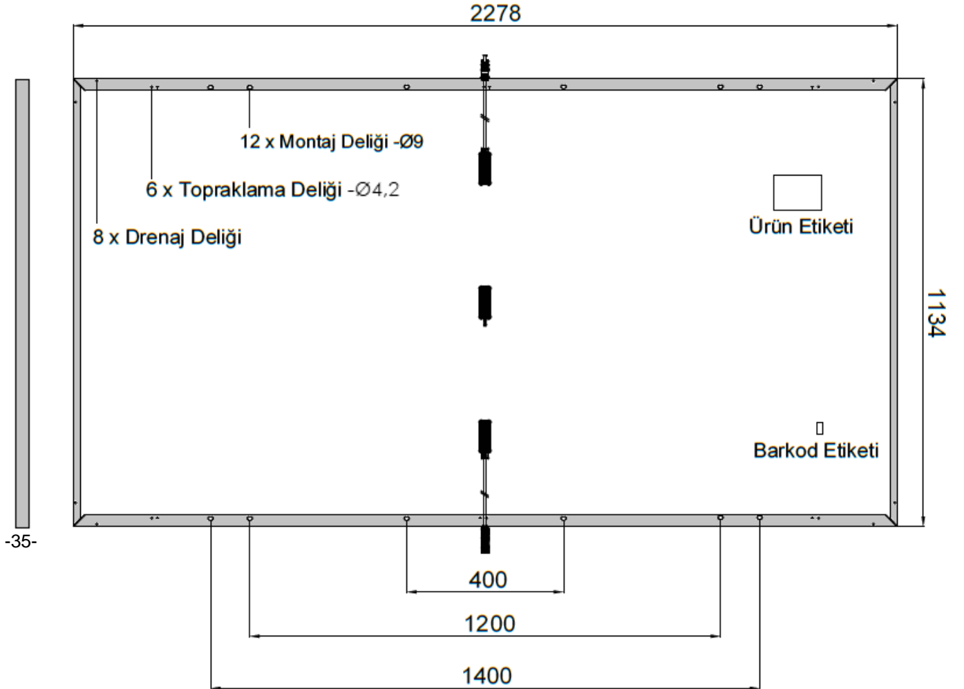
Şekil 1: SPE 540-144M/ SPE 545-144M/ SPE 550-144M panel arka görünümü ve boyutlandırması
