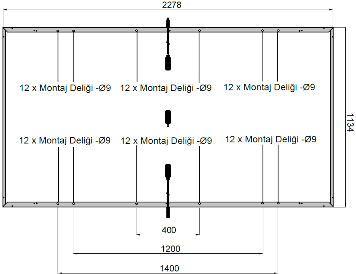
Şekil 2: Montaj deliklerine göre kurulum
