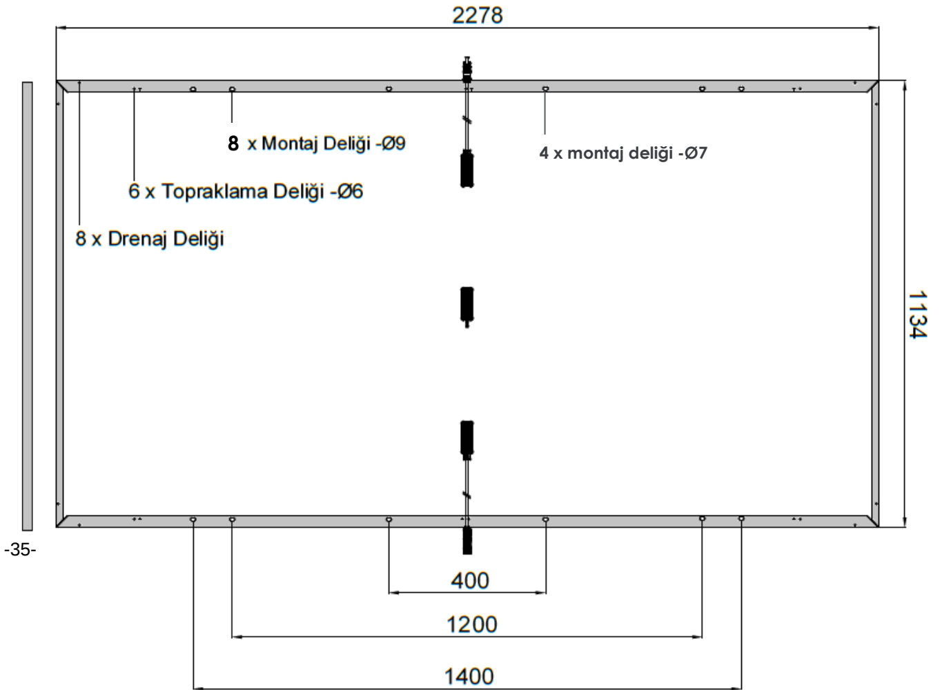
Şekil 1: SPE 540-144M/ SPE 545-144M/ SPE 550-144M/ SPE 545-144B/ SPE 550-144M panel boyutlandırması
