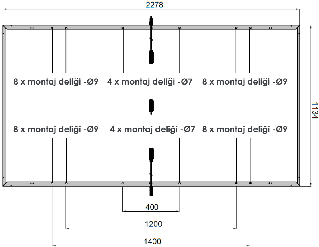
Şekil 3: SPE 540-144M/ SPE 545-144M/ SPE 550-144M / SPE 545-144B/ SPE 550-144B panel montaj delikleri
