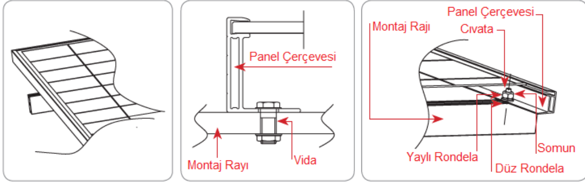
Şekil 2: Montaj deliklerine göre kurulum
